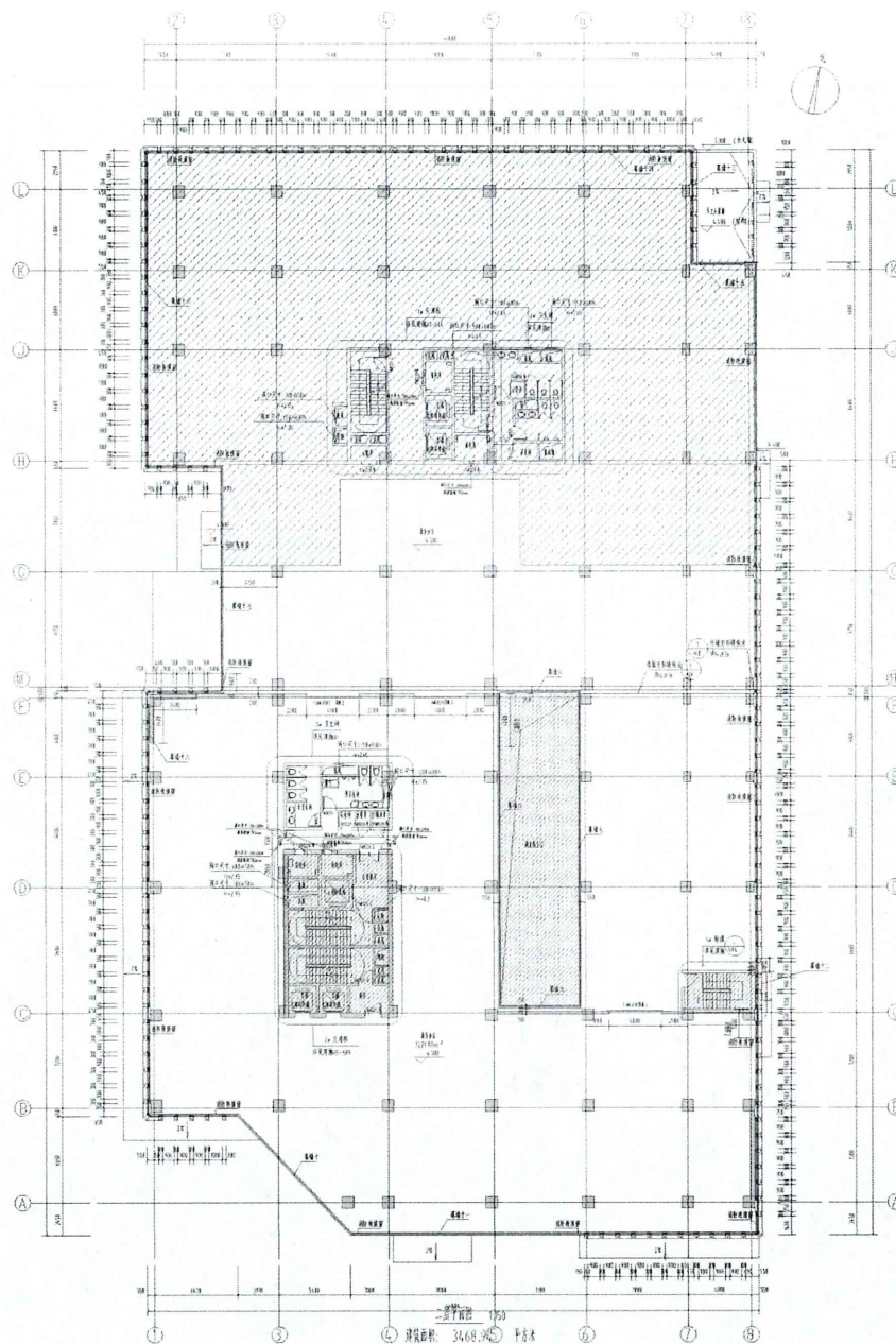
二层平面图 1:100
