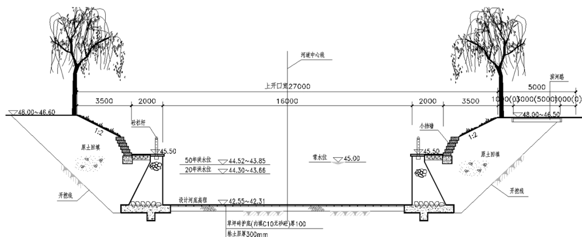
图 4-1 现状河道横断面图
