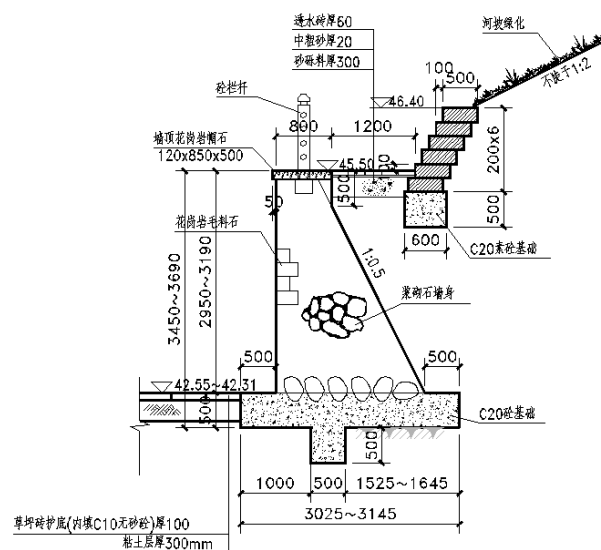
图 4-2 现状挡墙结构图
