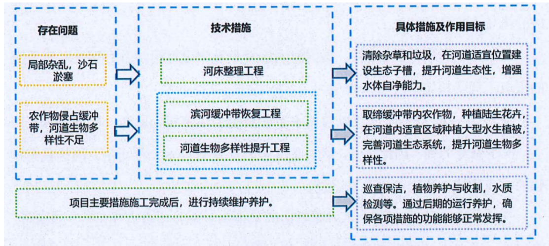
图 6-2 北庄河道生态措施技术路线图
