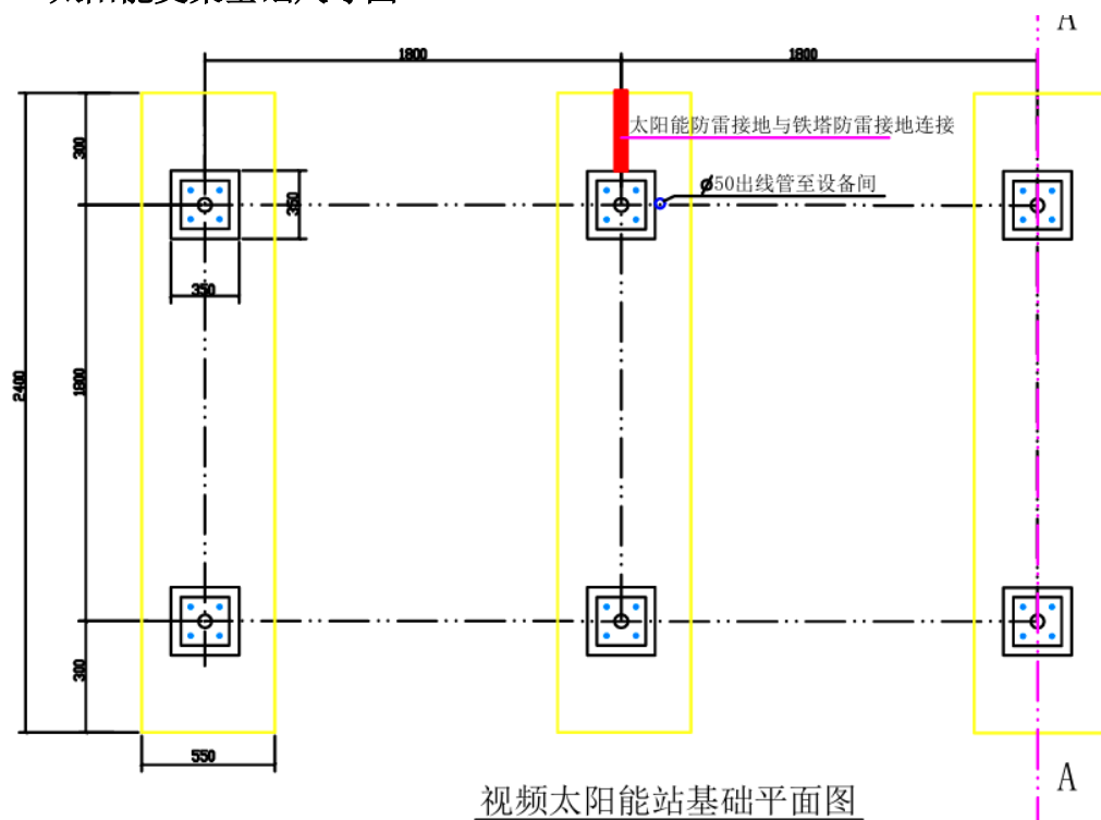
太阳能支架基础尺寸图
