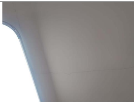
图4.1-19 9单元601屋面板板底裂缝
