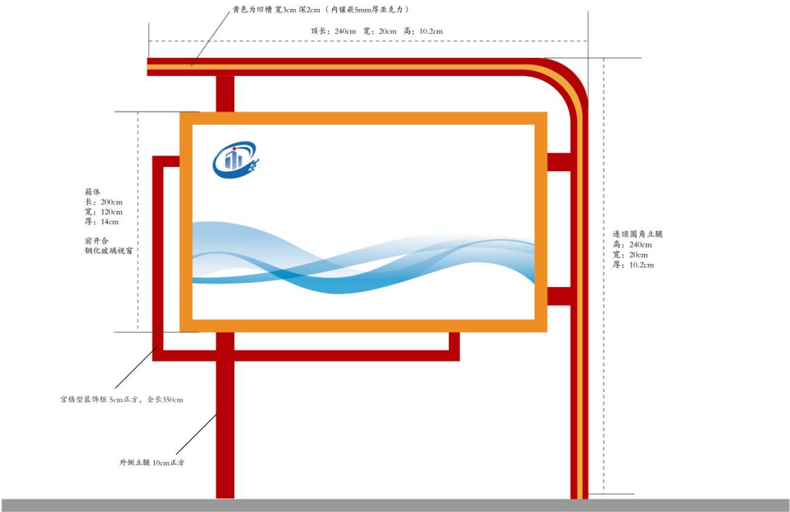
立式宣传栏造型设计图
