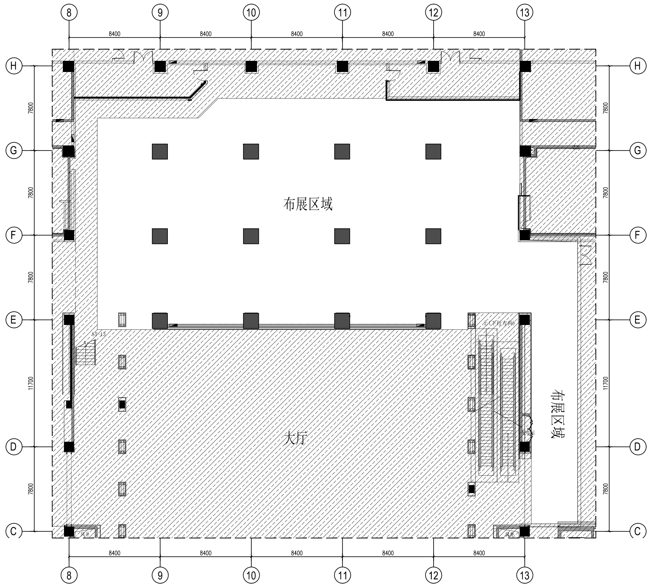
一层平面图
