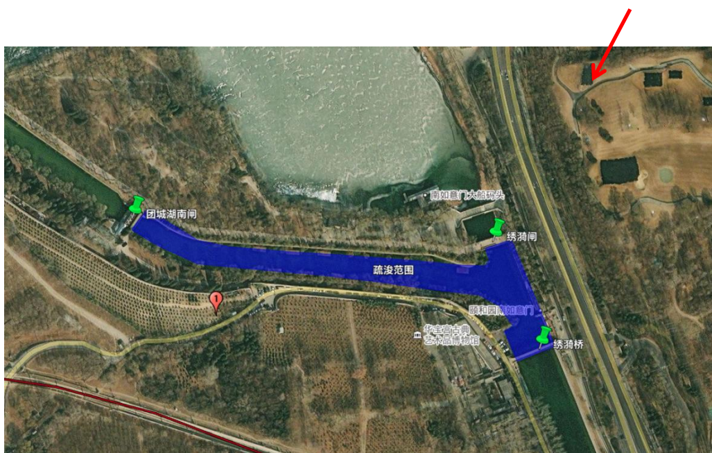
图 6 疏浚范围示意图（昆玉河（团城湖南闸-绣漪桥））
