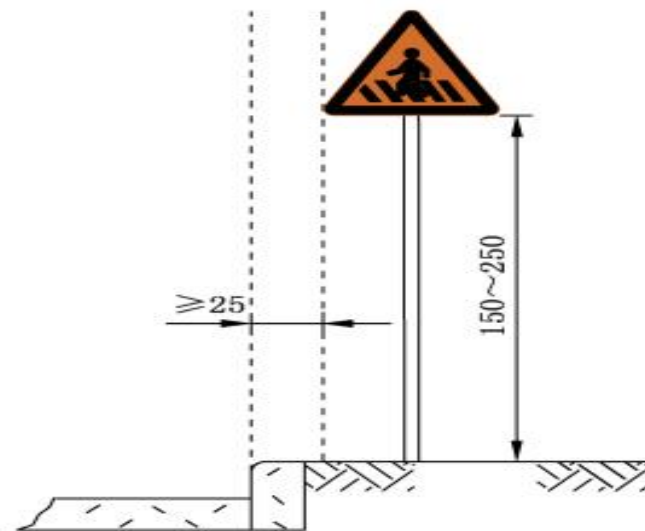
a) 单柱式
