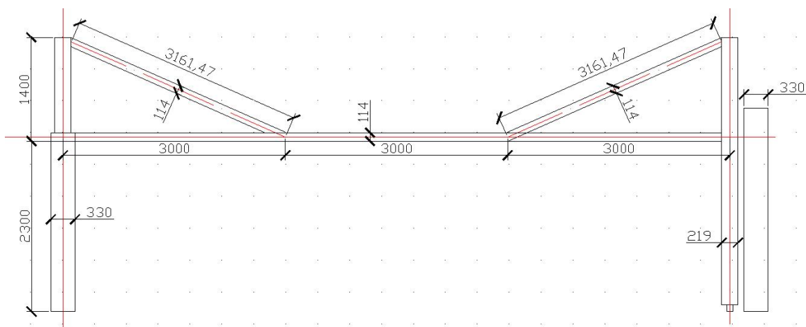
改造后限高杆
