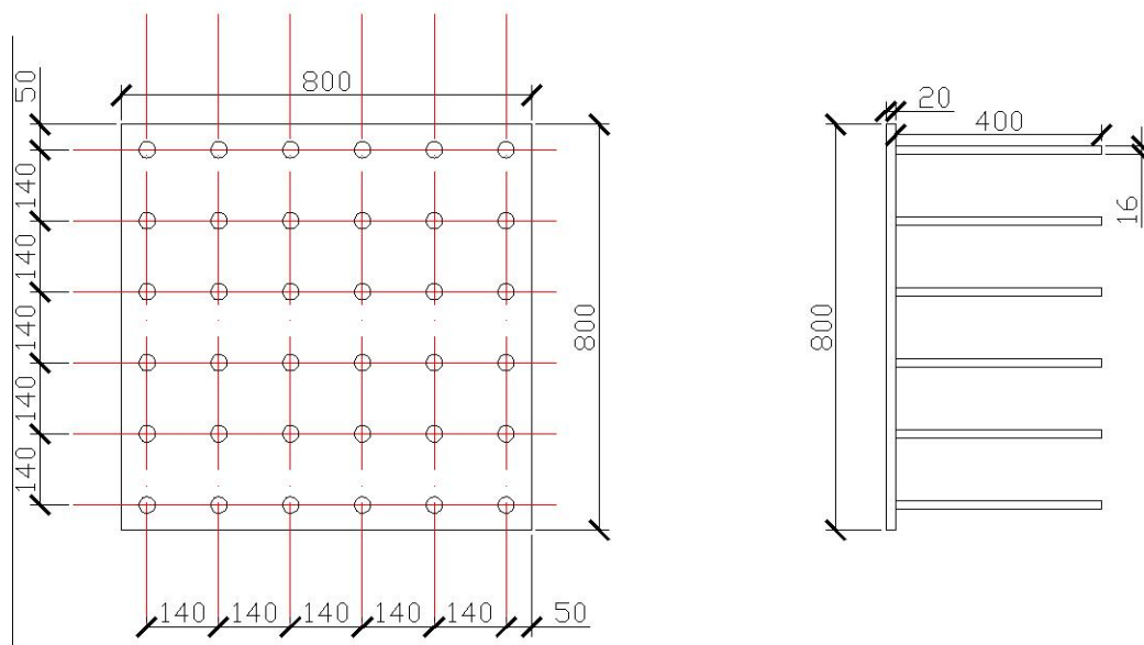
预埋件详图
