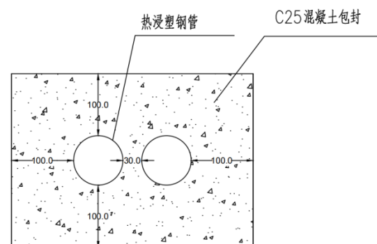
过路钢管混凝土包封横断面示意图
