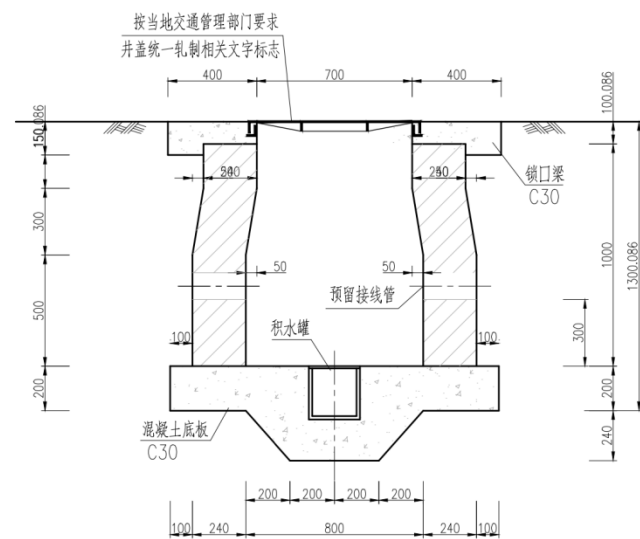
手孔井剖面图
