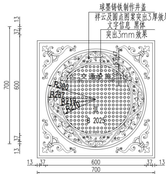
方框圆井盖 700*700mm 圆直径600mm
