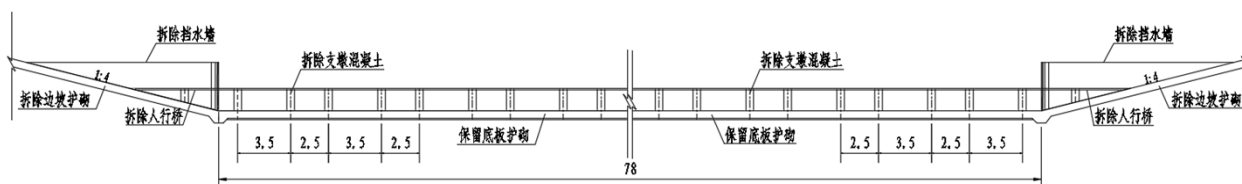
图 2-3 闸室拆除断面示意图（垂直水流方向）
