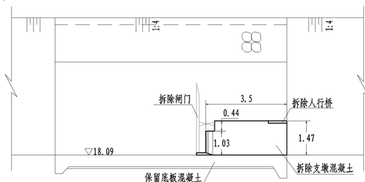
图 2-2 闸室拆除断面示意图（顺水流方向）
