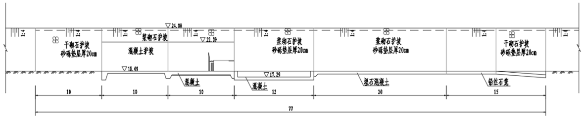
图 2-1 苇沟拦河闸顺水流向断面图
