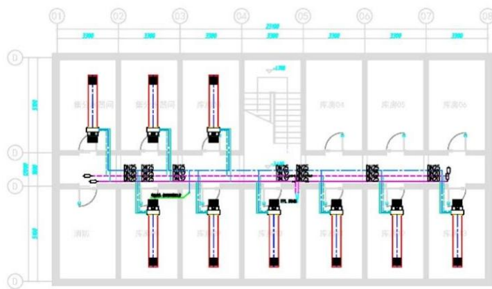
负一层风盘布置平面示意图
