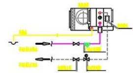
风机盘管水路接法示意图
