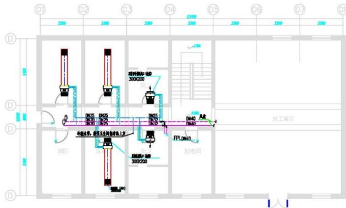
一层风盘布置平面示意图
