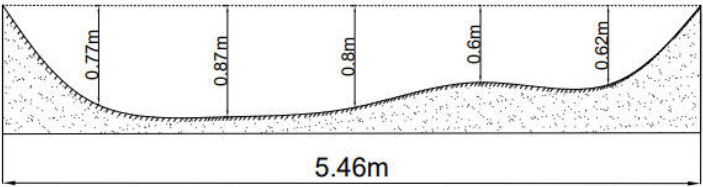
图 2 洪水断面示意图
