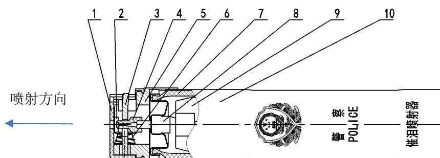
图1 横喷型催泪喷射器结构示意图
