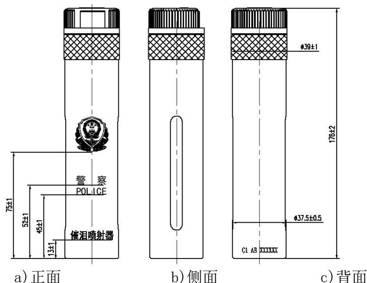
图 3 C1 催泪喷射器外形尺寸示意图 单位为毫米
