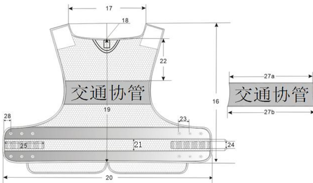
图 2a 反光背心成品尺寸测量方法
