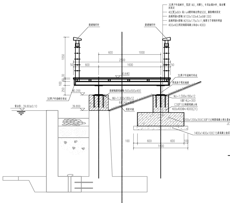
图 5-9 雍和宫桥下游新建栈道做法
