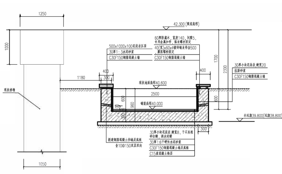
图 5-13 建材桥桥下下挖做法
