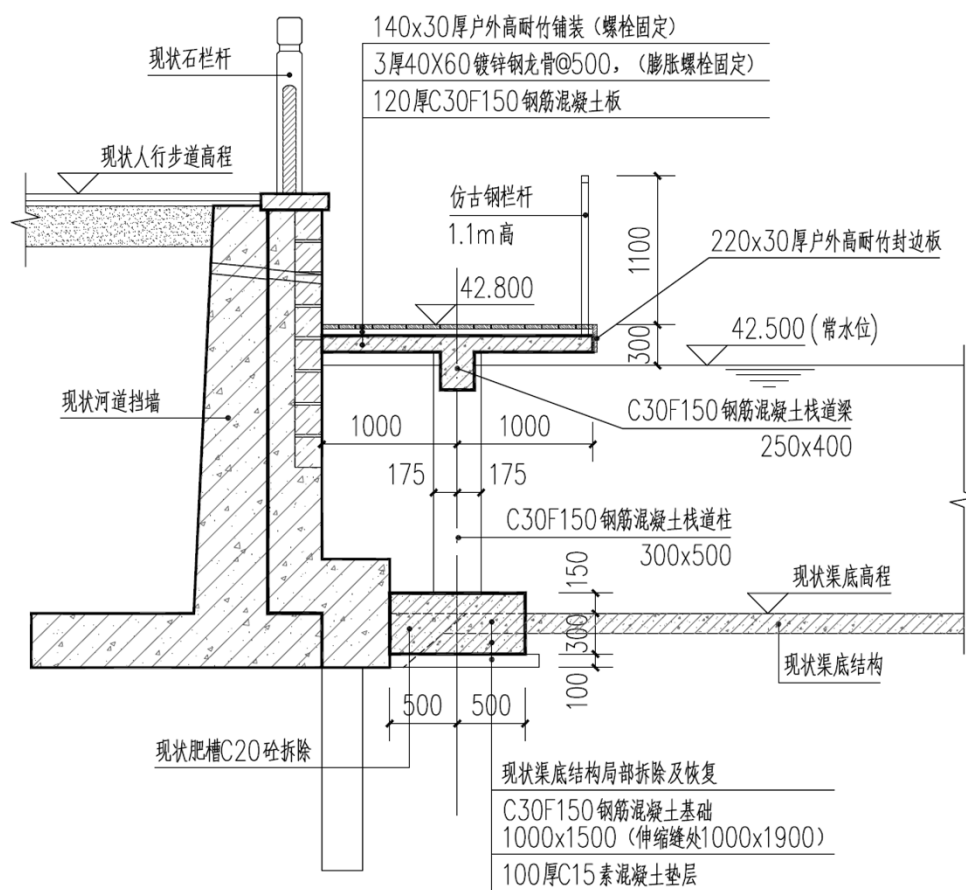
图 5-4 德胜门桥栈道做法 (3) 主要工程量
