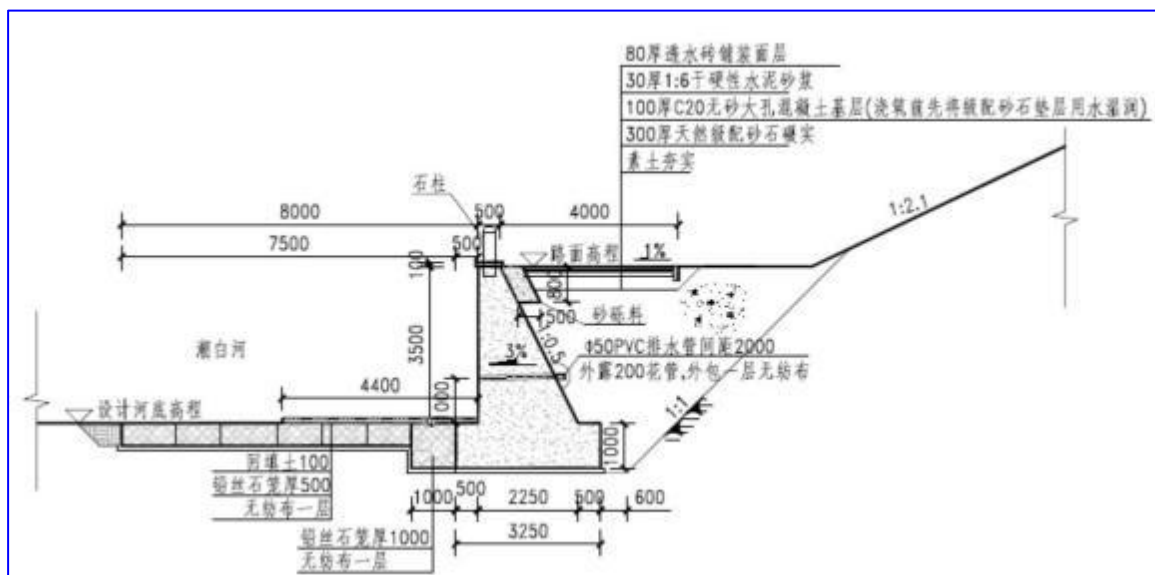
俸伯桥下游右岸挡墙修复断面
