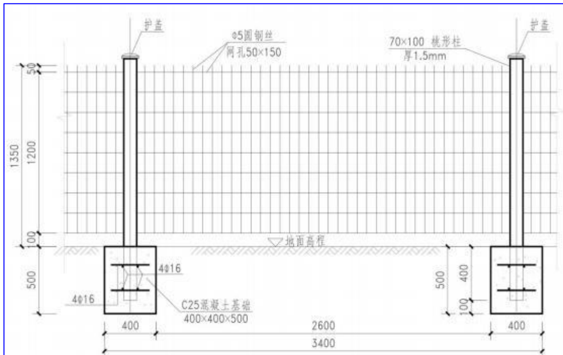
向阳闸下游右岸跌水段护网断面
