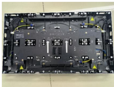
图 2-3 箱体外观检查
