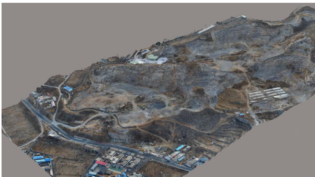
金大正+盛强建材厂治理区三维模型 图 2-6 治理区三维模型成果示意
