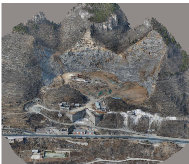
檀木港石灰厂治理区三维模型
