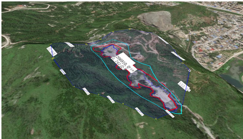
图 3-2 振兴石材厂治理区汇水面积图
