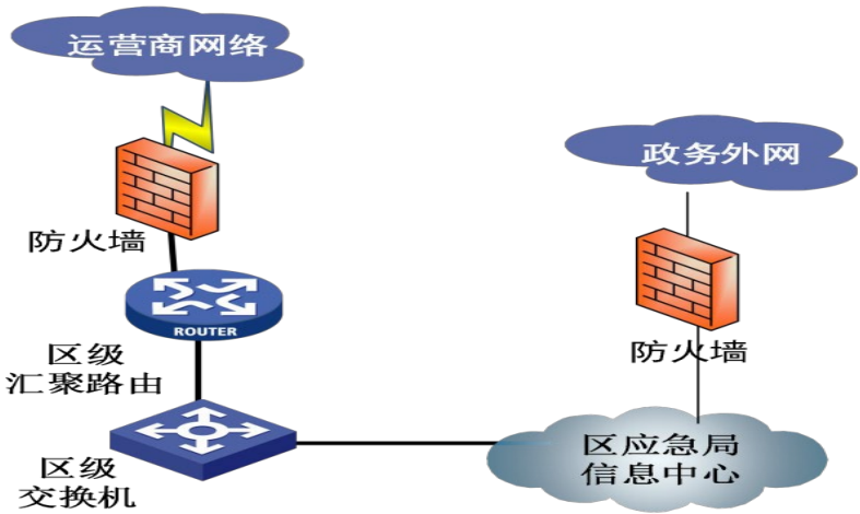
图 区应急管理局网络拓扑（接入部分）
