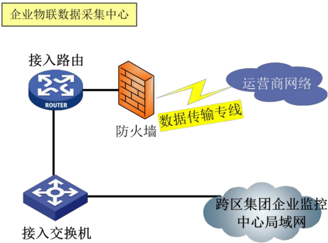
图 跨区域集团网络拓扑（接入部分）
