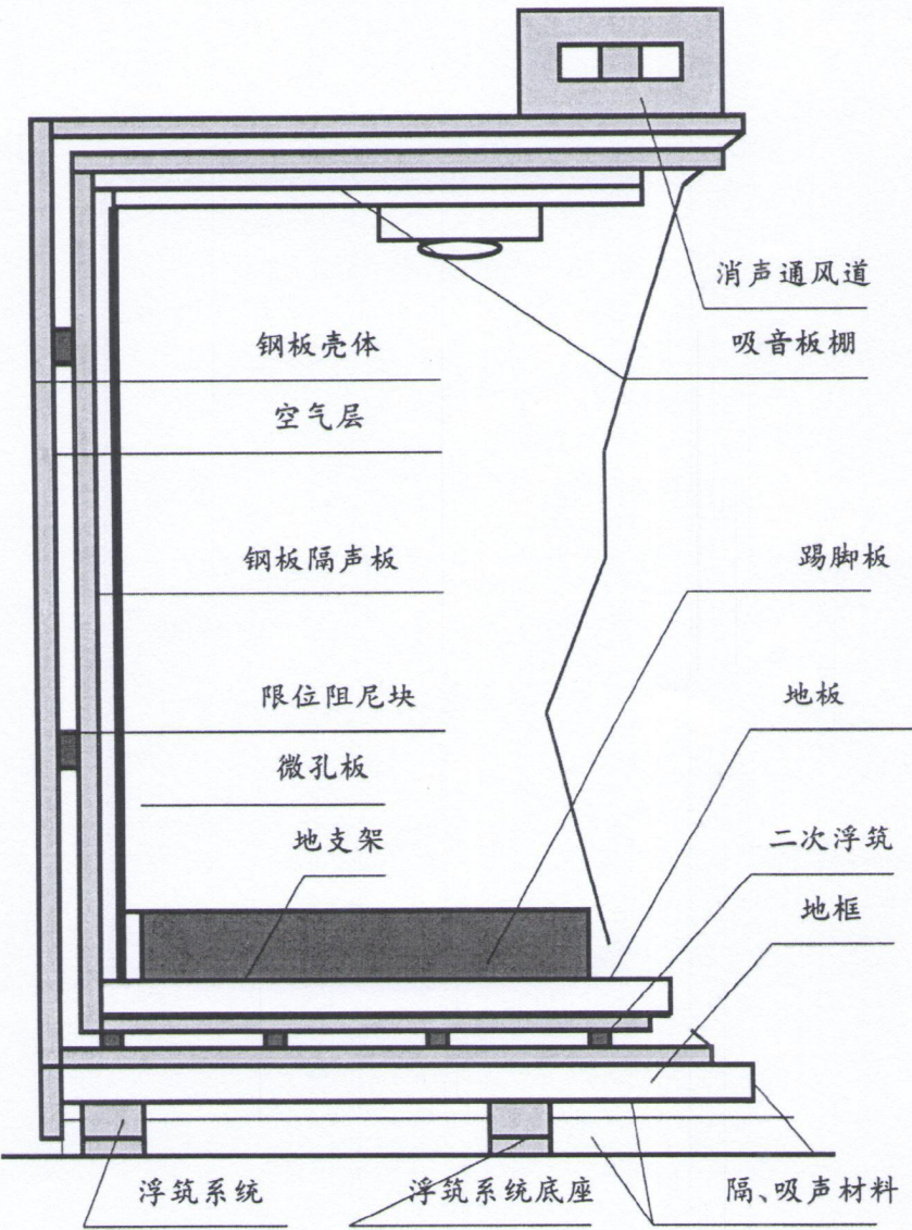
150 厚双层钢板纯音测听室结构图
